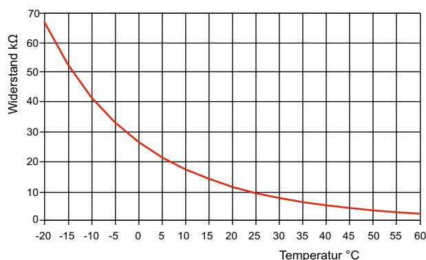
Abb. 7.1: Fühlerkennlinie NTC-10
