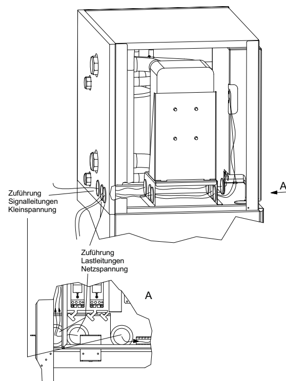
Abb. 7.3: Kabeleinföhrung Schaltkasten
